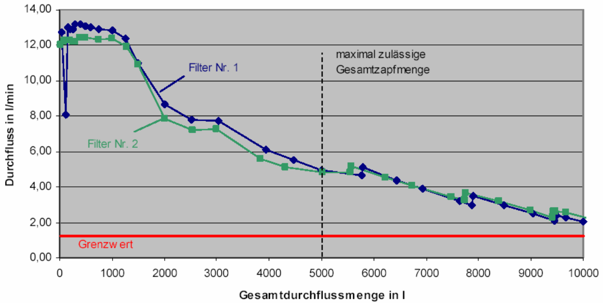
Carbonit Trinkwasserfilter mit Filterkartusche NFP Clario Durchfluss in Abhängigkeit von der Gesamtdurchflussmenge Lifetest vom April 04
