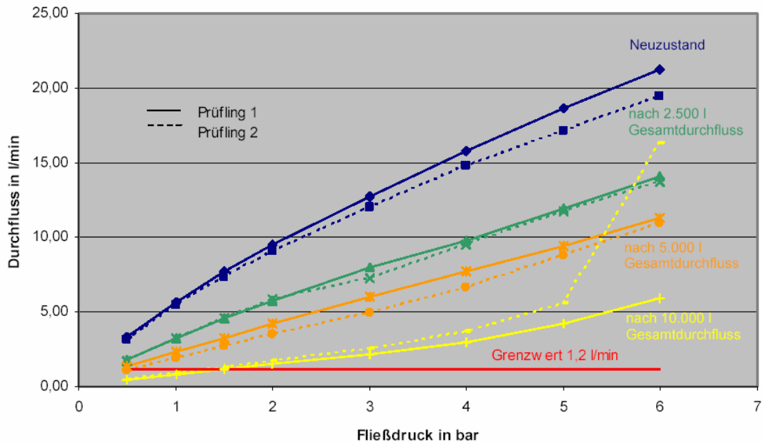
Carbonit Trinkwasserfilter mit Filterkartusche NFP Clario Durchfluss in Abhängigkeit vom Fließdruck Lifetest vom April 04
